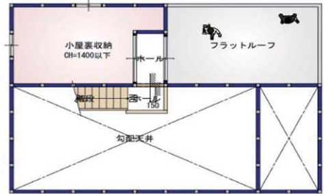
小屋裏PH平面図
