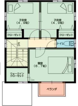
2階平面図
